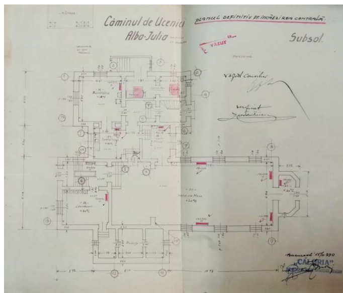
Căminul de Ucenici din Alba Iulia Proiect pentru plan subsol, cu instalații de încălzire, calorifere. dos. 197/1929
