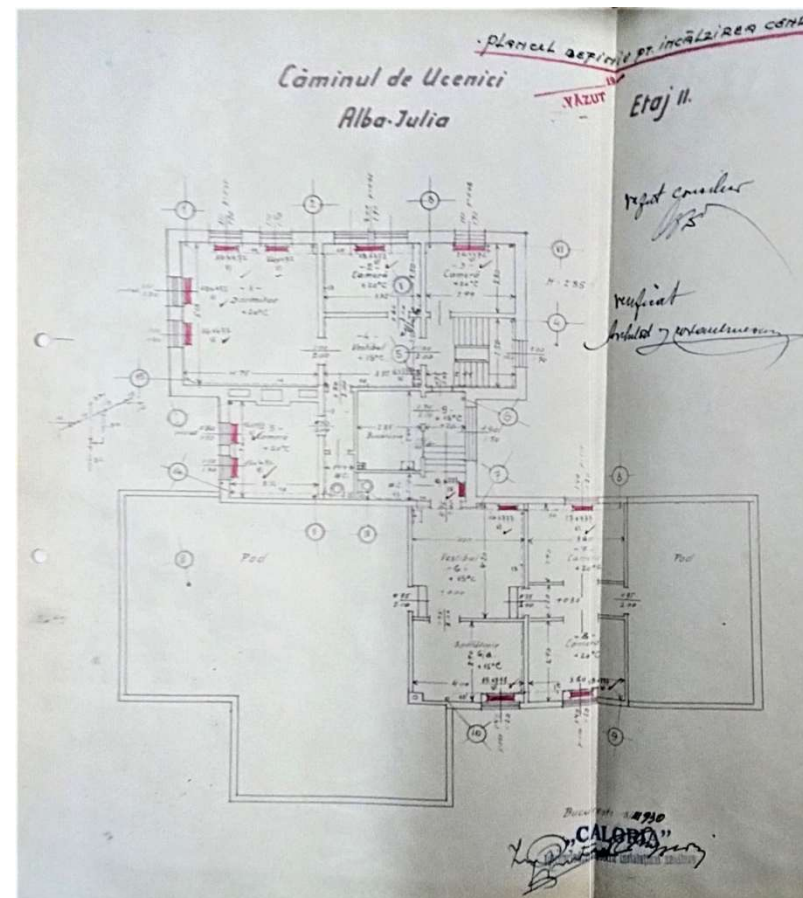
Căminul de Ucenici din Alba Iulia Proiect pentru planul etajului al II-lea, cu instalații de încălzire, calorifere. dos. 197/1929
