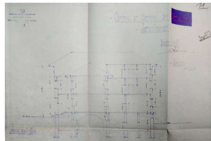
Căminul de Ucenici din Alba Iulia Proiect pentru secțiune, semnat de arhitectul Tașcu Ciulli
