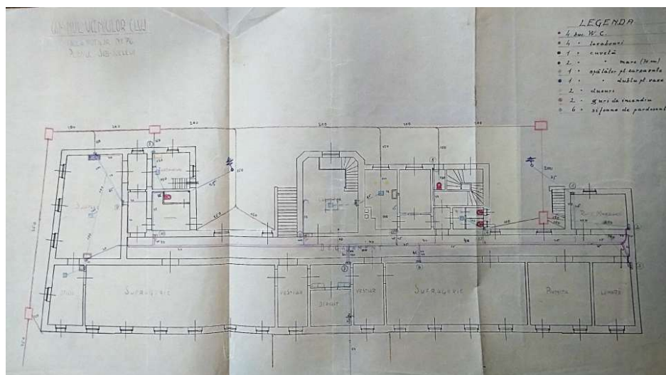
Căminul de Ucenici nr. 1 Cluj, planul subsol pentru instalații dos. 84/1928
