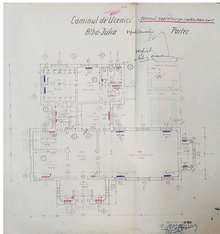
Căminul de Ucenici din Alba Iulia Proiect pentru plan demisol, cu instalații de încălzire, calorifere. dos. 197/1929 Â
