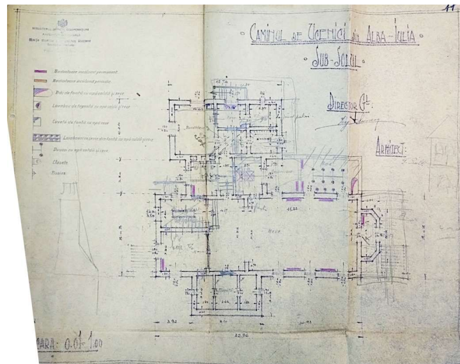
Căminul de Ucenici din Alba Iulia Proiect pentru plan subsol, cu instalațiile de încălzire, calorifere, instalații sanitare, dorecturi și schițe, semnat de arhitectul Tașcu Ciulli dos. 197/1929
