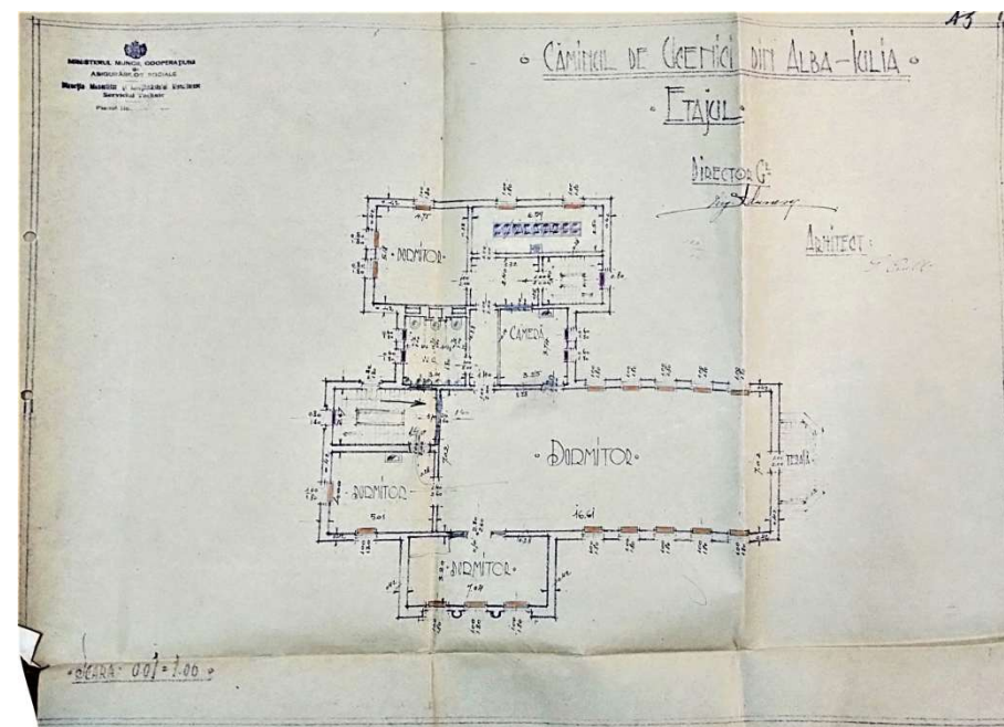
Căminul de Ucenici din Alba Iulia. Proiect pentru plan subsol, cu instalațiile de încălzire, calorifere, semnat de arhitectul Tașcu Ciulli
